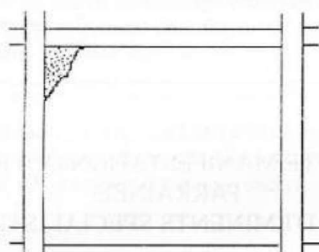
Ecrasement de l'angle comprimé
