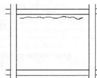
Ecrasement du mur (mauvaise qualité de la maçonnerie sous les poutres)
